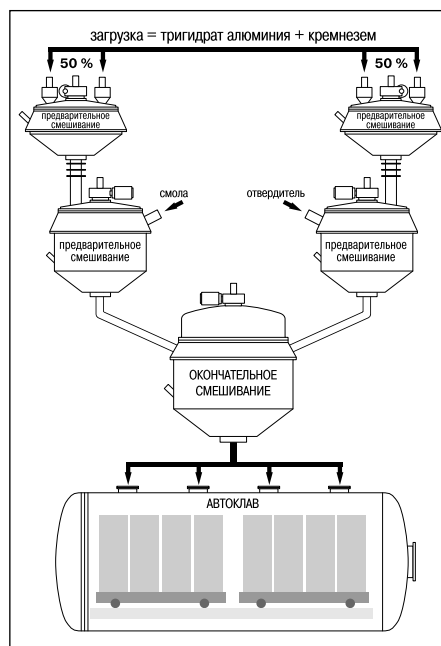
Схема процесса вакуумной заливки
